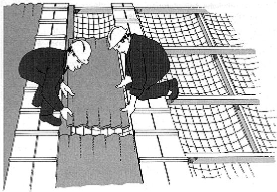
Bild 15: Lauf- und Arbeitsstege auf nicht durchsturzsicheren Bauteilen
