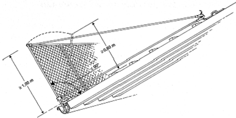
Bild 12: Dachschutzwand
